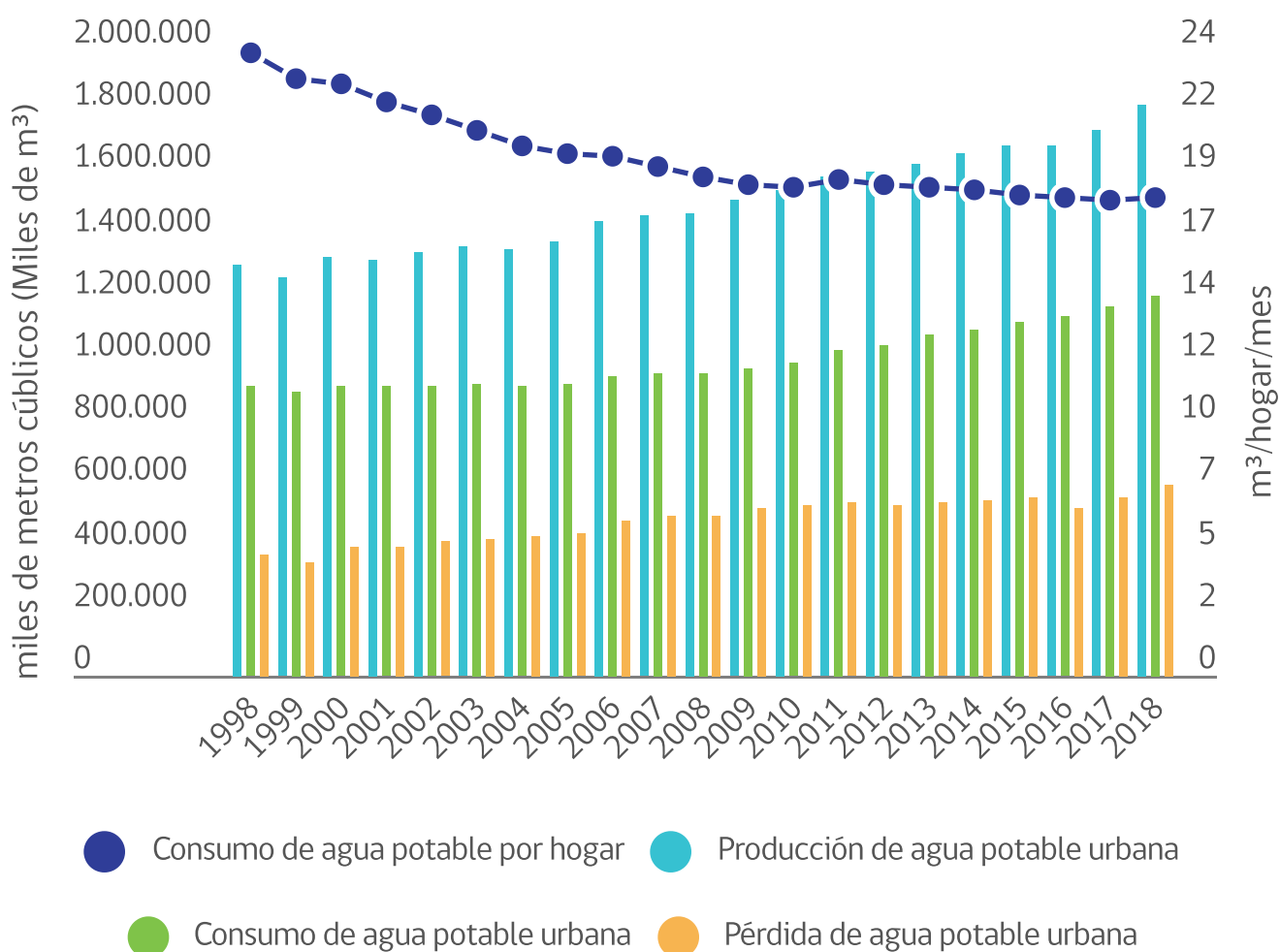
Producción, consumo y pérdida nacional de agua potable, 1998-2018
