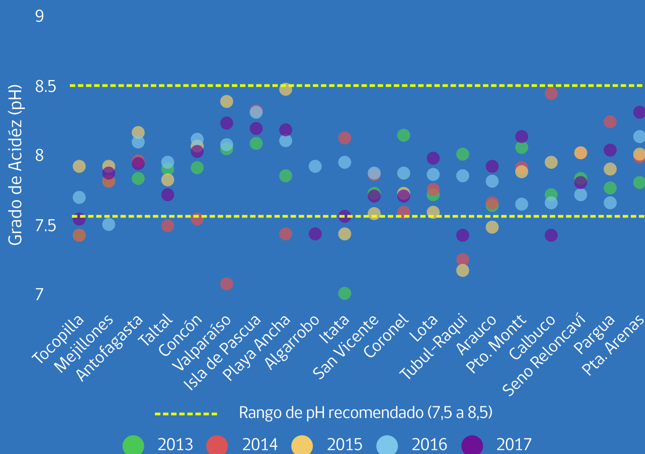
pH medio anual medido en estaciones marítimas representativas, 2013-2017
