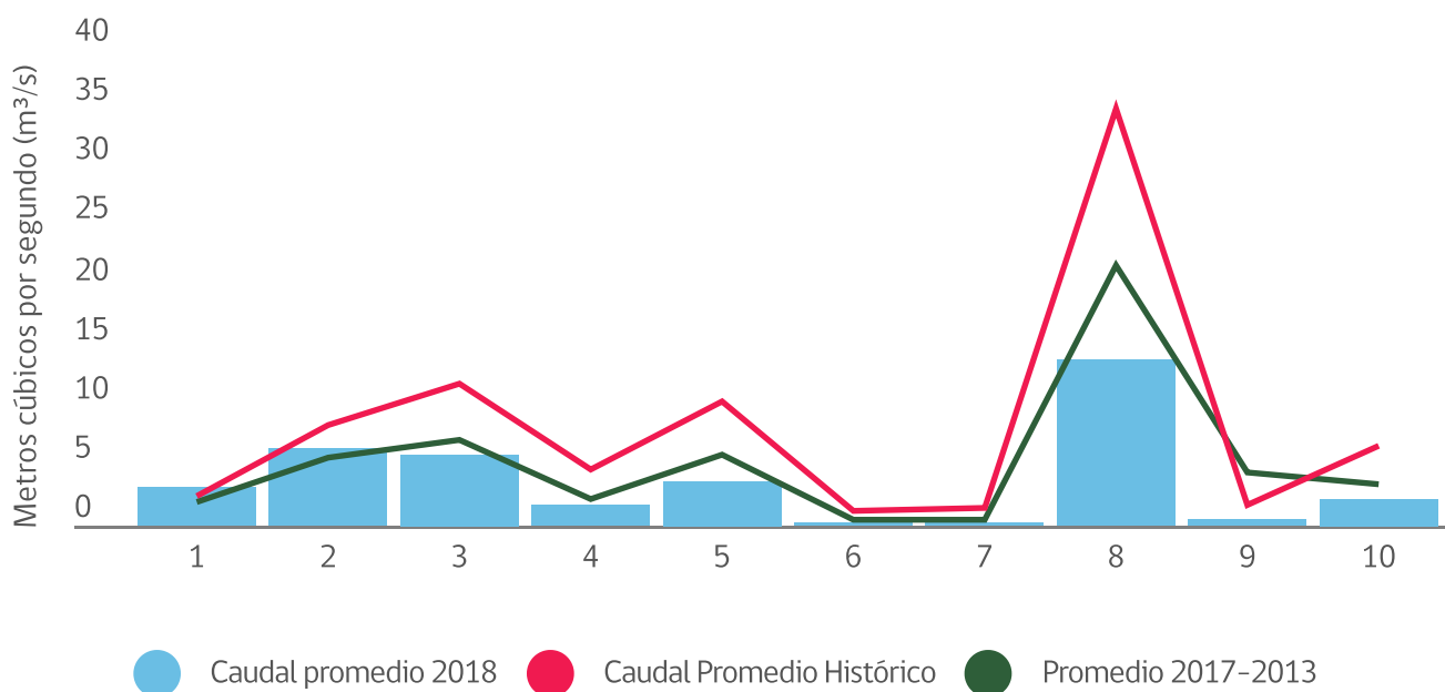
Variación de caudales zona norte, 2018
