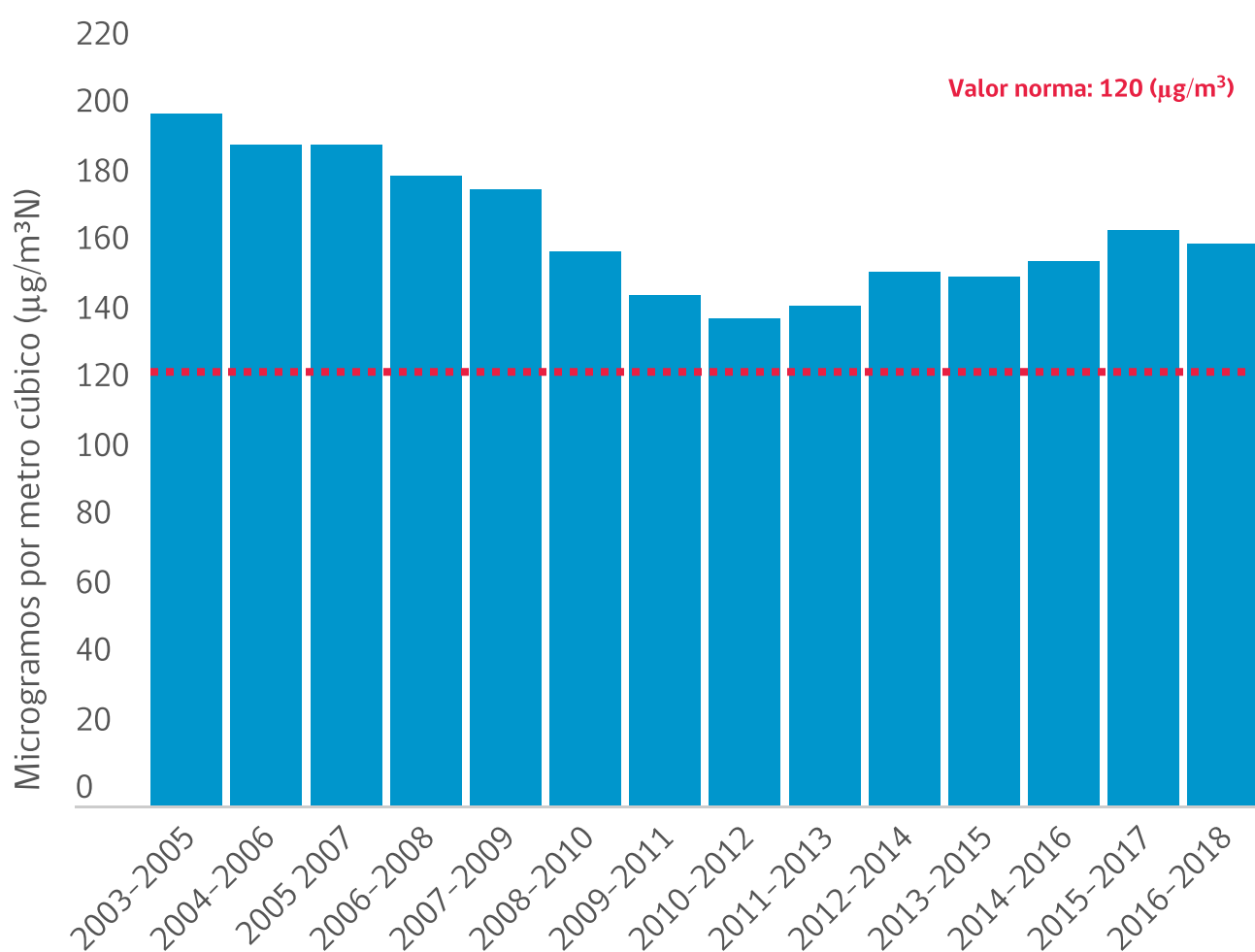
Evolución trianual del Percentil 99 de las concentraciones de ozono ( \text{O}_3 ) en estaciones de monitoreo de la Región Metropolitana, 2003–2018
