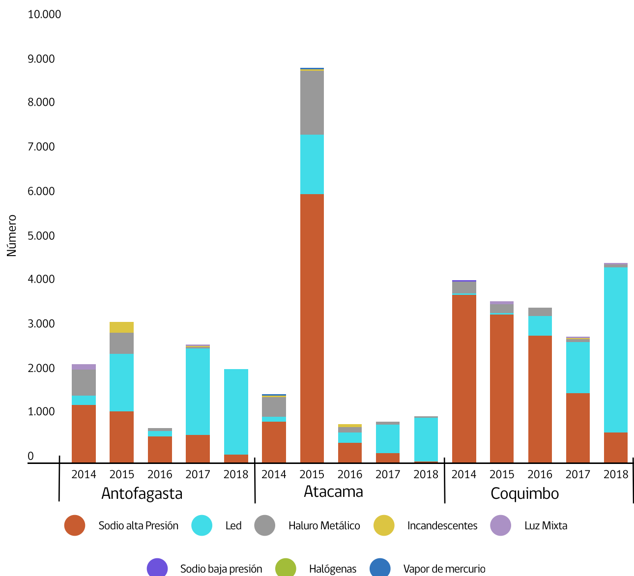
Luminarias nuevas en las regiones de Antofagasta, Atacama y Coquimbo, según tecnología, 2014-2018
