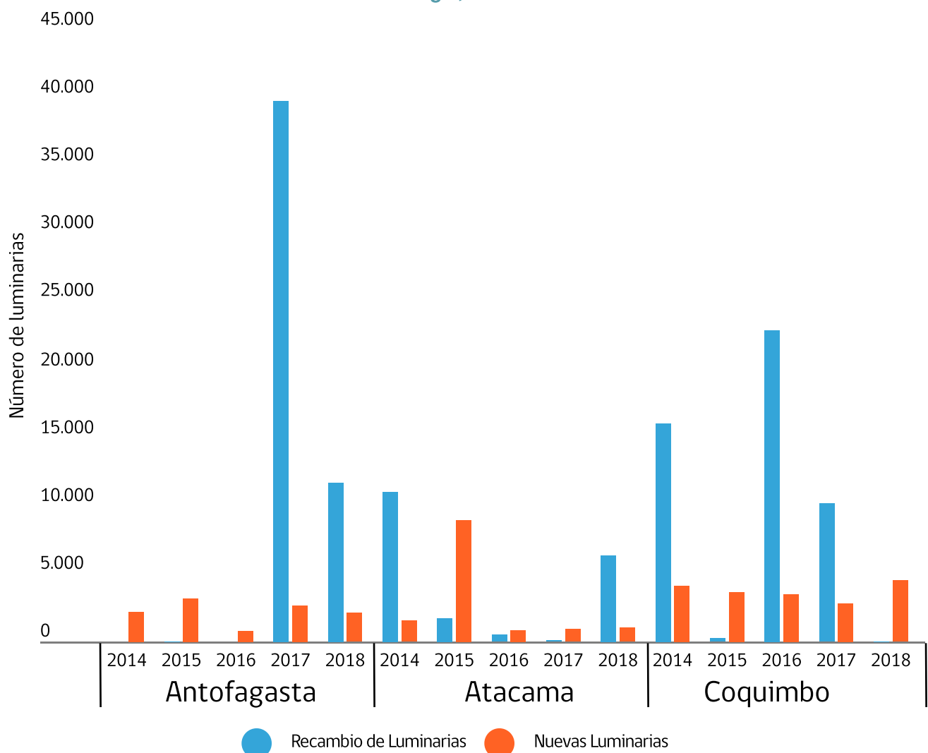
Recambio y luminarias nuevas en las regiones de Antofagasta, Atacama y Coquimbo, según tecnología, 2014-2018
