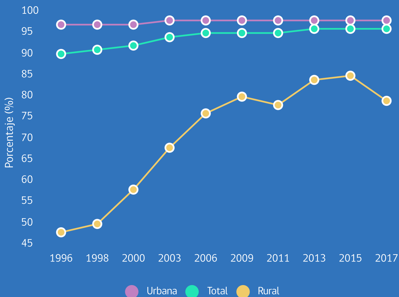
Proporción de la población que utiliza servicios de agua potable de manera segura, 1996-2017
