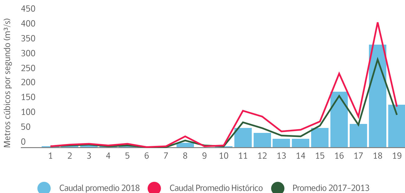
Variación de caudales, 2018
