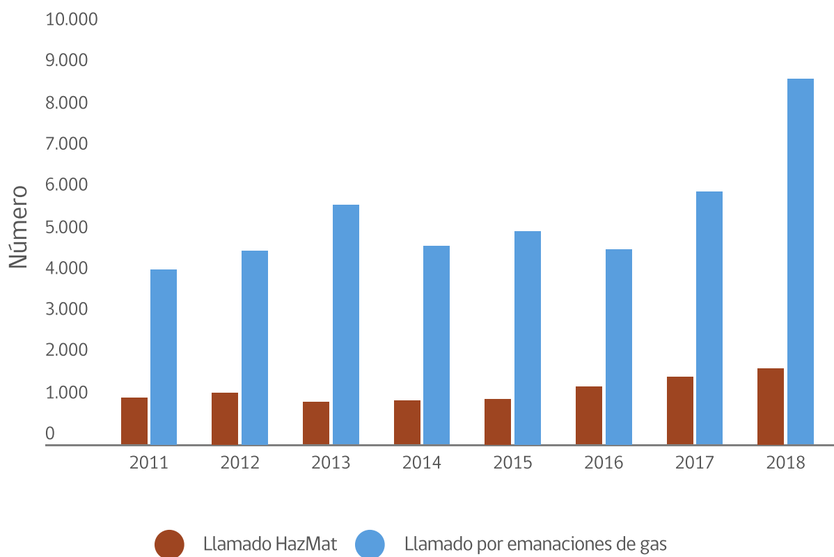
Emergencias con materiales peligrosos a nivel nacional, 2011-2018
