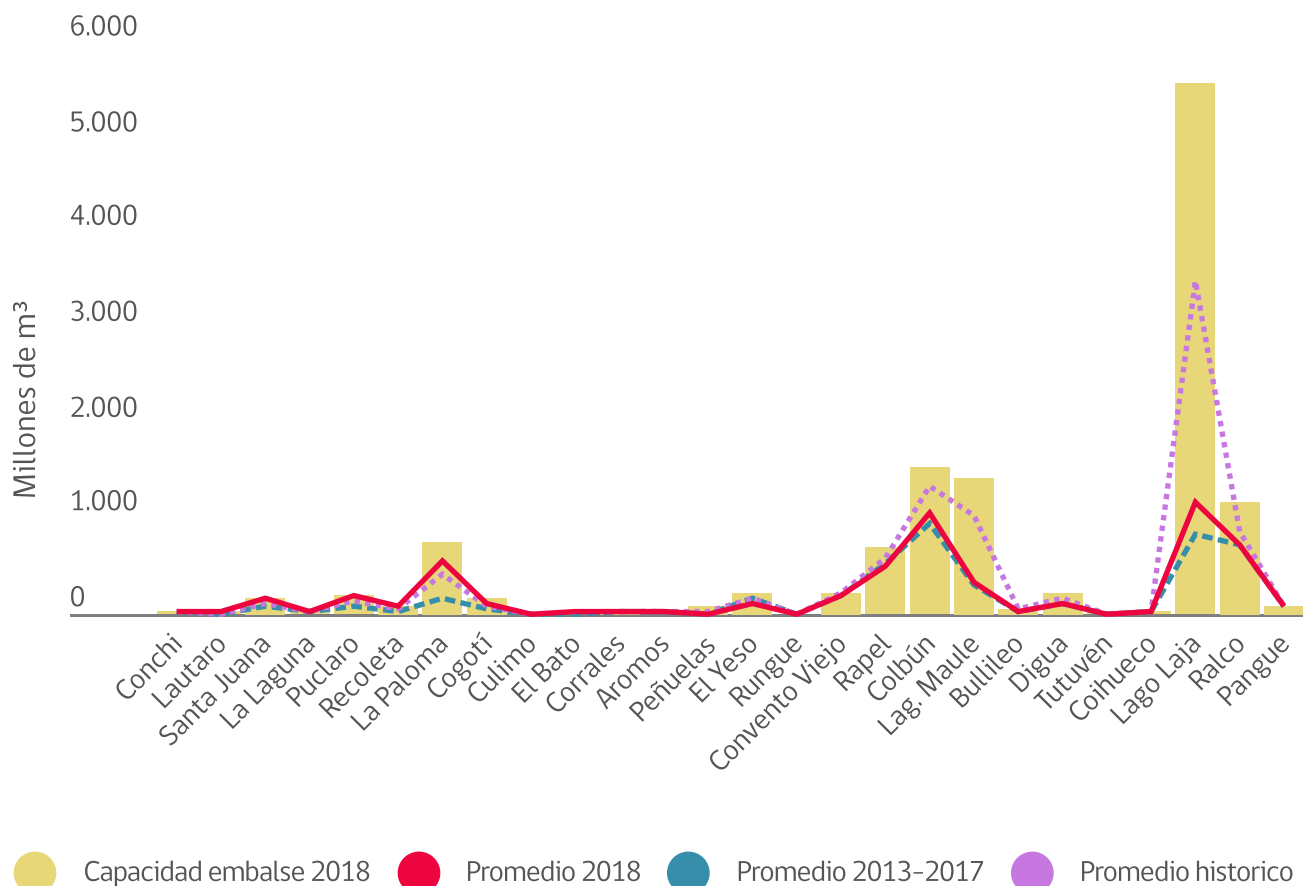
Volúmenes de agua embalsada, 2018
