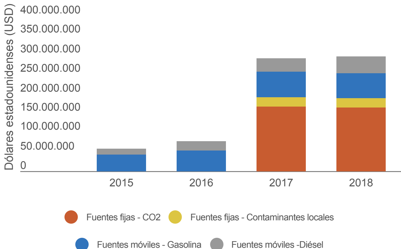
Recaudación de impuestos verdes sobre fuentes móviles y fijas, 2015-2018
