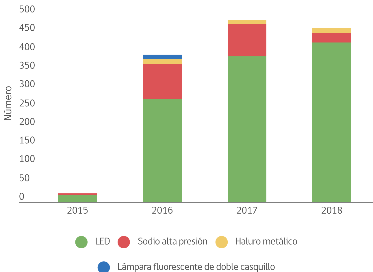
Certificaciones otorgadas según tipo de tecnología de luminarias, 2015-2018
